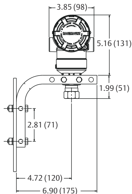
Illustration 21 : Configurations de montage typiques du Rosemount 2051T avec support de montage en option
