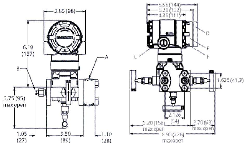
Illustration 11 : Rosemount 2051C Coplanar avec manifold intégré traditionnel à trois vannes Rosemount 305
