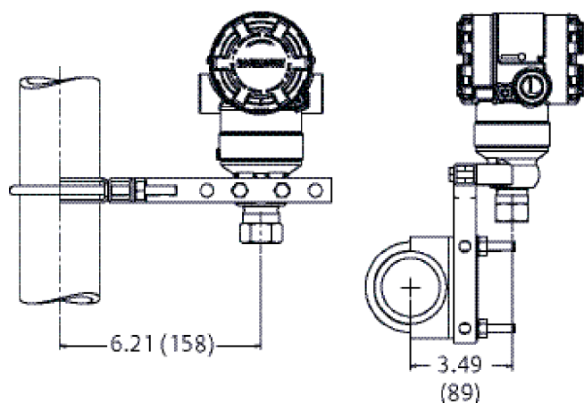
Illustration 21 : Configurations de montage typiques du Rosemount 2051T avec support de montage en option
