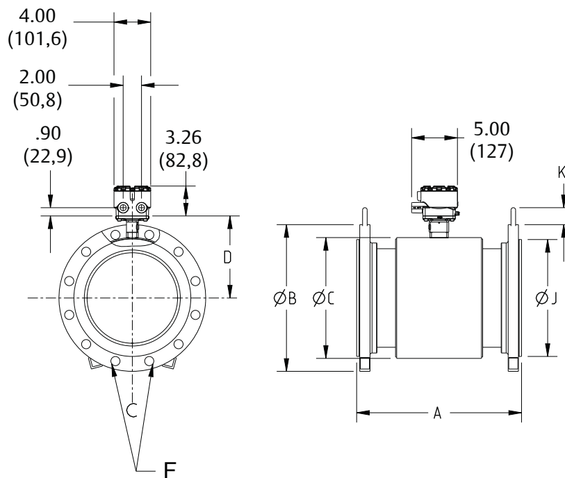
Illustration 11 : Capteur à bride à face surélevée de 75 à 1 200 mm
