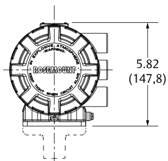
Illustration 8 : Transmetteur à montage mural avec couvercle standard
