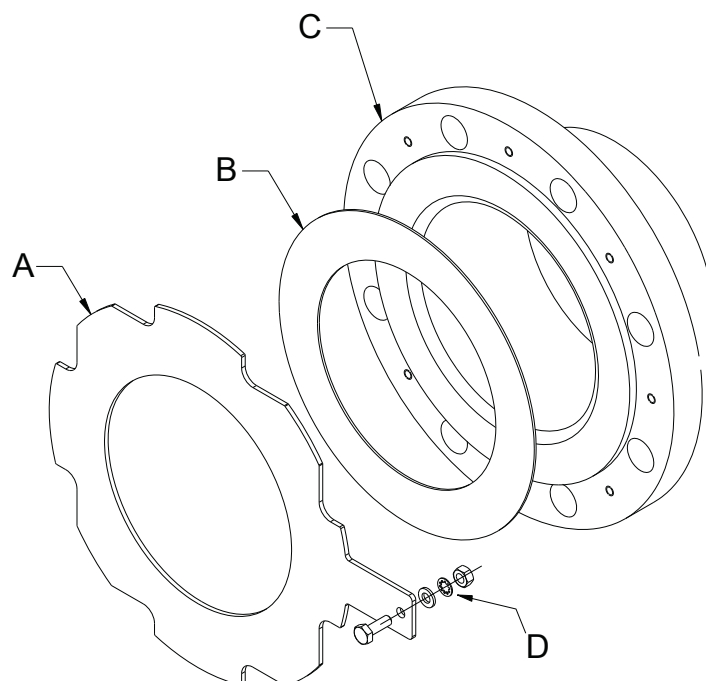
Illustration 13 : Anneau de mise à la masse du capteur à bride de 15 à 1 200 mm
