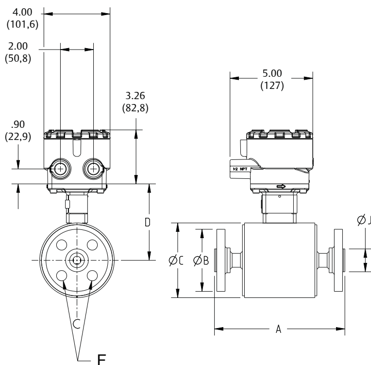
Illustration 10 : Capteur à bride à face surélevée de 15 à 65 mm
