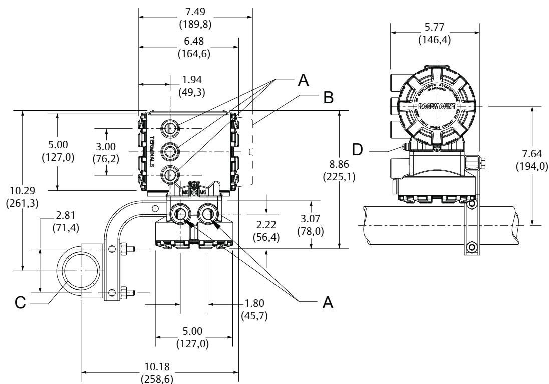
Illustration 6 : Transmetteur à montage mural déporté
