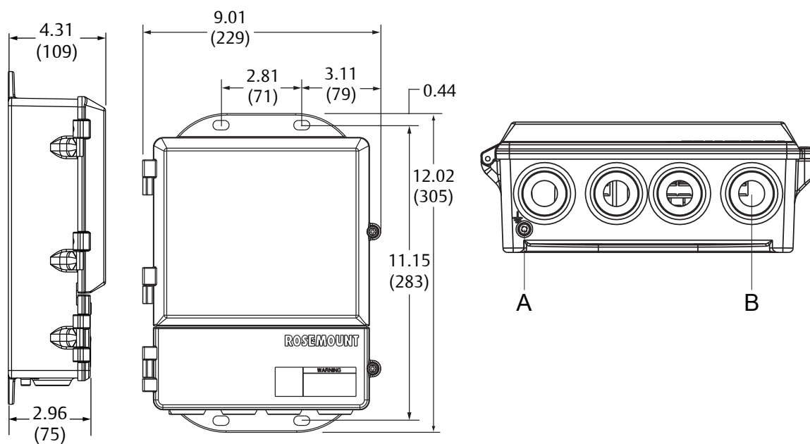
Illustration 8 : Transmetteur à montage mural avec couvercle standard
